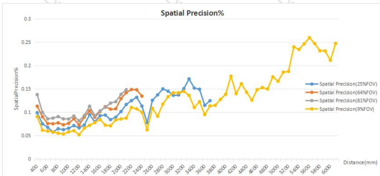
图 5-1-1 Gemini 435Le 空间相对精度
