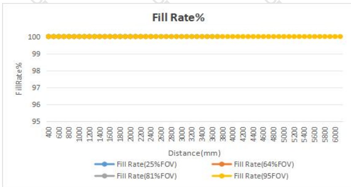
图 5-1-3 Gemini 435Le 深度填充率
