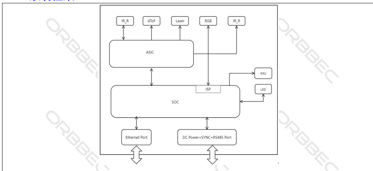
图 4-3-1 Gemini 435Le 相机系统框图
