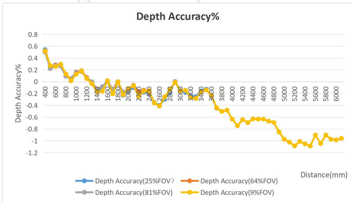
图 5-1-4 Gemini 435Le 深度绝对精度
