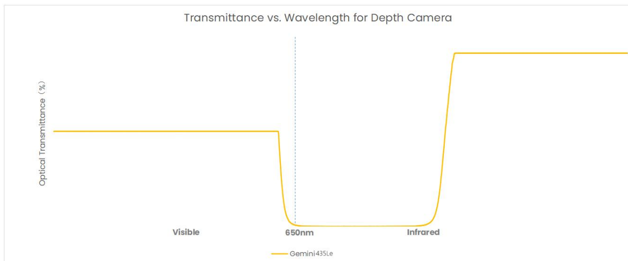
图 3-4-7 深度相机不同波段透过率一览图
