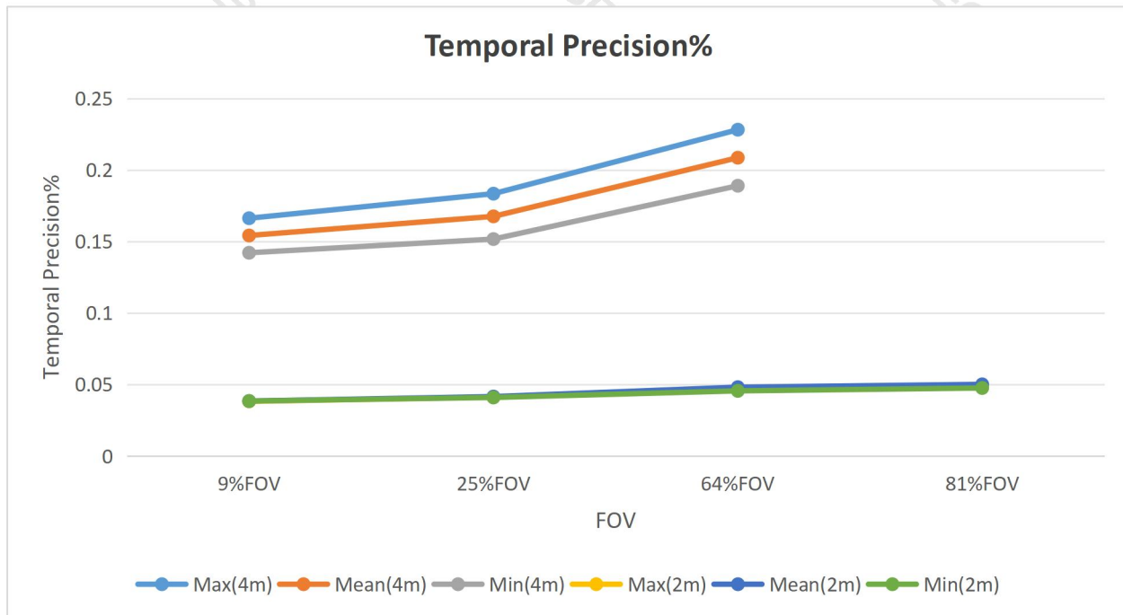
图 5-1-2 Gemini 435Le 时间相对精度参考图
